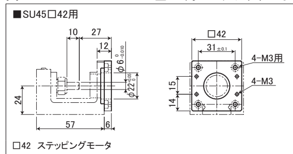
☒ : SU45×50-MB42 ☐ 42用モータブラケット
