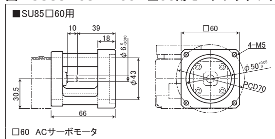
☒ : SU85×65-MB60 ☐ 60用モータブラケット
