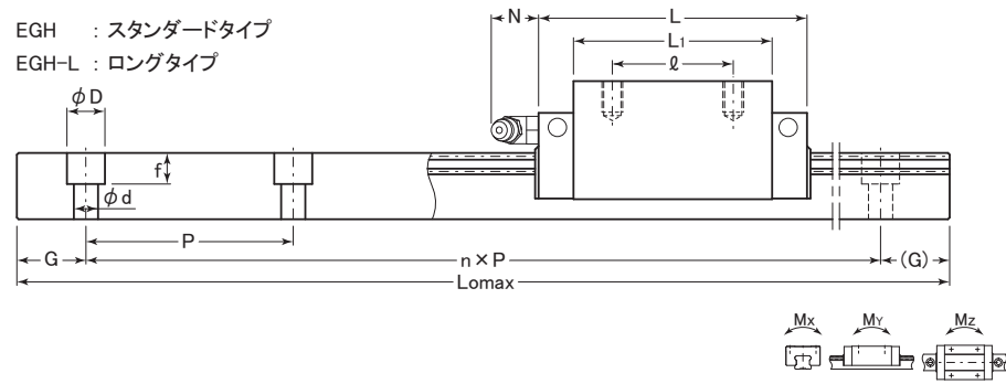
単位 : mm
